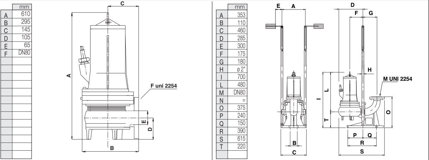
Con dispositivo di accoppiamento - With coupling foot - Avec dispositif de raccordement
